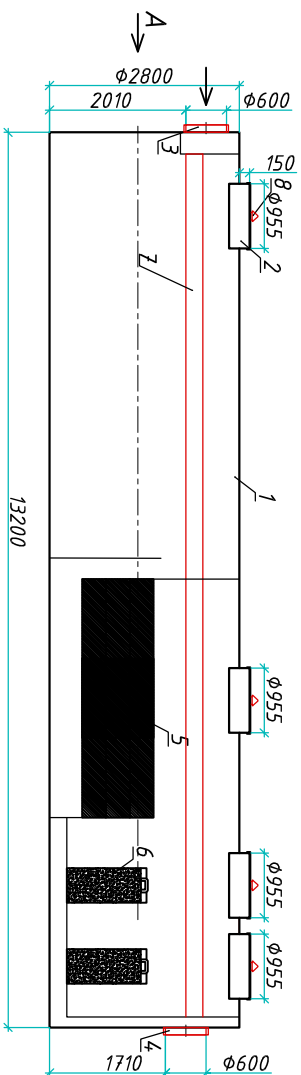
Разрез 1-1
