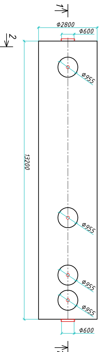
Вид сверху
