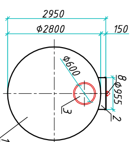
Вид А
